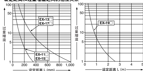
设定距离和过量增益之间的相互关系
