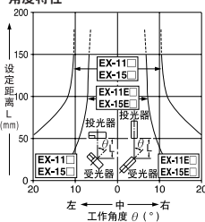
角度特性
