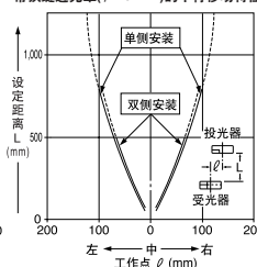
带狭缝透光罩( \phi 1.5\text{mm} )的平行移动特性
