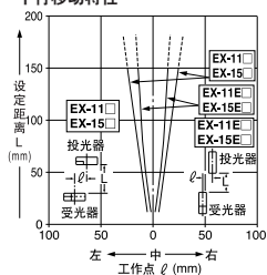
平行移动特性
