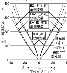
带狭缝透光罩( \phi 1.2\text{mm} )的平行移动特性
