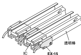
检测薄片
