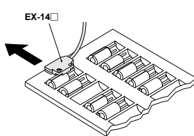
检测托盘上电容器的缺少
