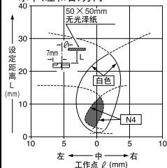
EX-14 限定反射型
